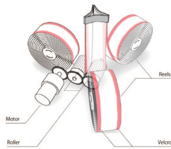
グランプリ作品プラン(アクチュエーター部分)
