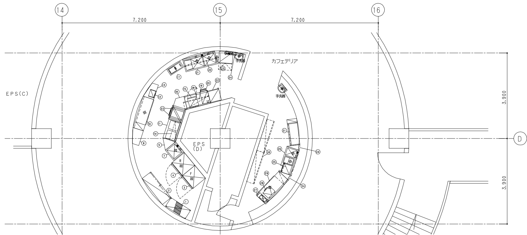
2階 カフェテリア厨房詳細図 S=1/50
